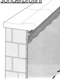
Sonderprofil II
